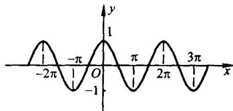
余弦函数
