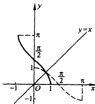
反余弦函数
