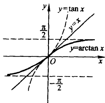
反正切函数
