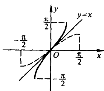
反正弦函数
