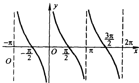
余切函数
