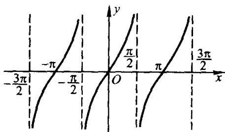
正切函数
