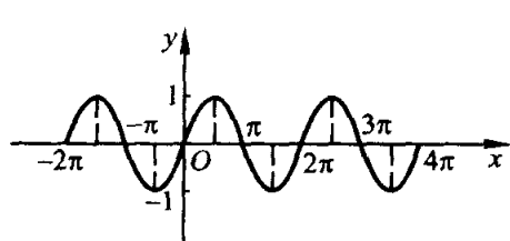
正弦函数
