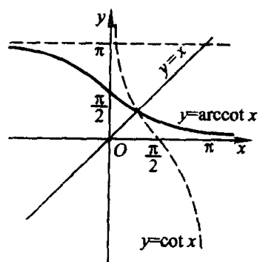
反余切函数
